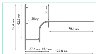
W30 DRIP EDGE
