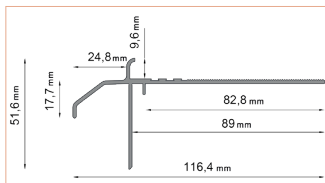
K20R DRIP EDGE
