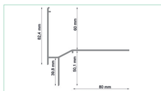
W60 DRIP EDGE
