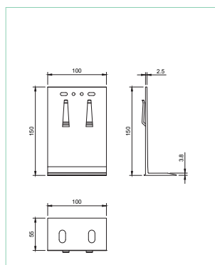
KONSOLA STAŁA 150x100x55
