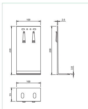
KONSOLA STAŁA 200x100x55
