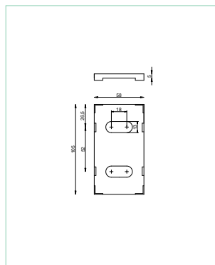
PRZEKŁADKA TERMICZNA DO KONSOLI STAŁEJ 105x58
