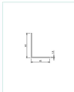
PROFIL KĄTOWY L 60x45
