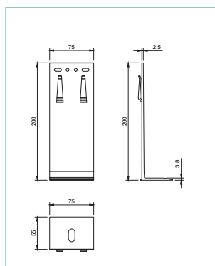
KONSOLA WIATROWA 200x75x55
