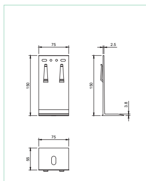
KONSOLA WIATROWA 150x75x55
