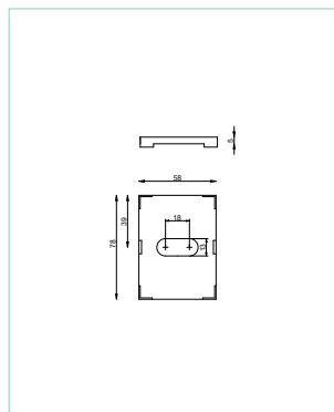
PRZEKŁADKA TERMICZNA DO KONSOLI WIATROWEJ 78x58
