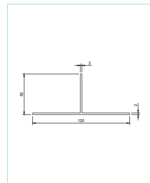
PROFIL TEOWY T 120x50
