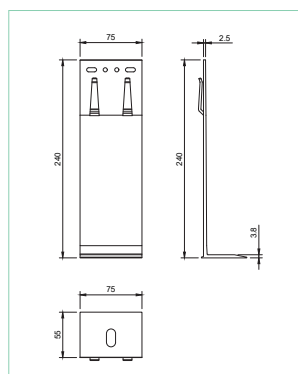
KONSOLA WIATROWA 240x75x55
