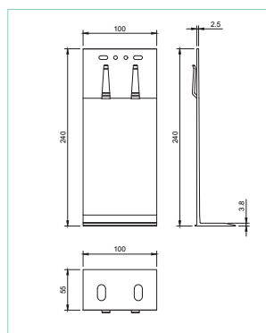
KONSOLA STAŁA 240x100x55
