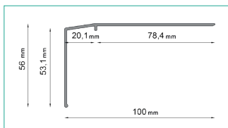
K301 DRIP EDGE
