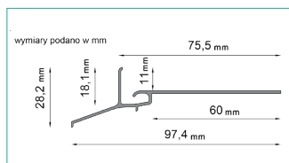
K102 DRIP EDGE
