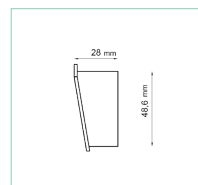
OPW20/OPW20R/OPW35 PLUS R+L WALL PROTECTION END CAPS
