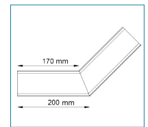
NAROŻNIK WEWNĘTRZNY RYNNY RK65 135
