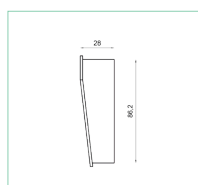
OPW30 ODBOJNIK PRZYŚCIENNY
