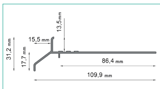
PROFIL PROSTY K30
