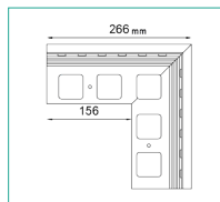
NZ K30/90 NAROŻNIK ZEWNĘTRZNY
