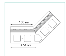
NW K30/135 NAROŻNIK WEWNĘTRZNY
