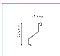
LK30 ŁĄCZNIK
