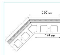
NZ K30/135 NAROŻNIK ZEWNĘTRZNY
