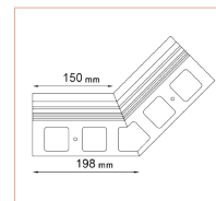
NW K20/135 NAROŻNIK WEWNĘTRZNY
