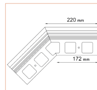
NZ K20/135 NAROŻNIK ZEWNĘTRZNY
