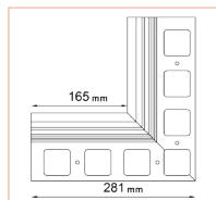
NW K20/90 NAROŻNIK WEWNĘTRZNY
