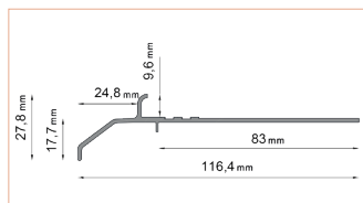
PROFIL PROSTY K20
