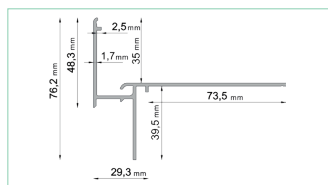
PROFIL PROSTY W35+
