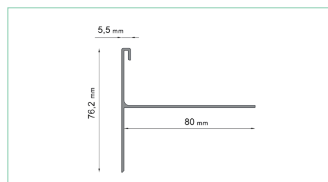
PROFIL BOCZNY W35B
