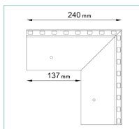
NZ W35+/90 NAROŻNIK ZEWNĘTRZNY
