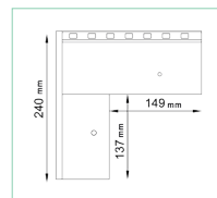
NAROŻNIK ŁĄCZĄCY W35+/W35B/90 LEWY
