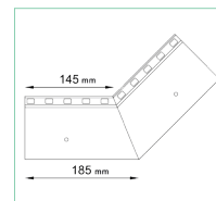
NW W35+/135 NAROŻNIK WEWNĘTRZNY
