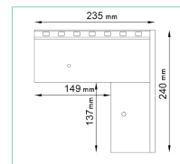
NAROŻNIK ŁĄCZĄCY W35+/W35B/90 PRAWY
