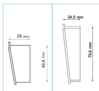
OPW35+ OPW35B ODBOJNIK PRZYŚCIENNY
