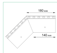
NZ W35+/135 NAROŻNIK ZEWNĘTRZNY
