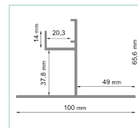
WSPORNIK PODSTOPNICY GÓRNY
