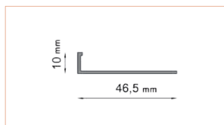
PROFIL SCHODOWY SZ10
