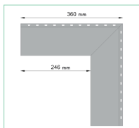
NAROŻNIK ZEWNĘTRZNY SCHODOWY SW 90 MAXI
