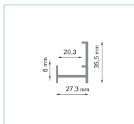
WSPORNIK SWD 6 cm
