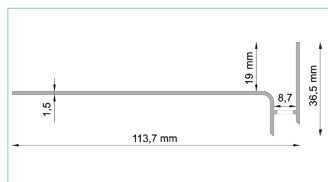
PROFIL SCHODOWY SW
