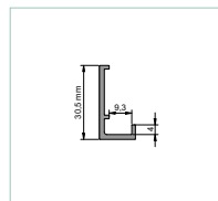
WSPORNIK SWD UKRYTY 6 cm
