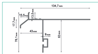
PROFIL OKAPOWY K40
