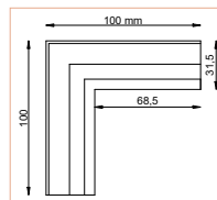
NAROŻNIK ŁĄCZNIKOWY K20/K20R
