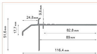
PROFIL OKAPOWY K20R
