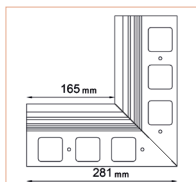
NAROŻNIK WEWNĘTRZNY K20 90
