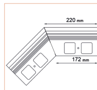
NAROŻNIK ZEWNĘTRZNY K20 135
