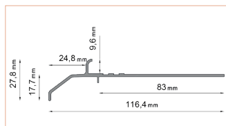
PROFIL OKAPOWY K20
