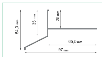
PROFIL OKAPOWY D25
