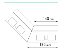
NAROŻNIK WEWNĘTRZNY D25 135
