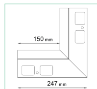
NAROŻNIK WEWNĘTRZNY D25 90
