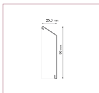
ZAKOŃCZENIA COKŁOWE OPC2 P+L
