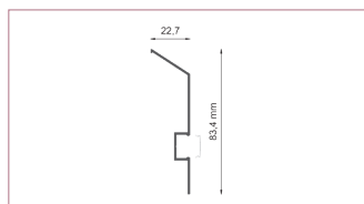
PROFIL COKŁOWY C2
