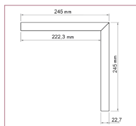
NAROŻNIK ZEWNĘTRZNY COKŁOWY C2 90 MAXI
