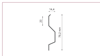
PROFIL COKŁOWY C1
