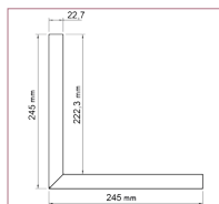
NAROŻNIK WEWNĘTRZNY COKŁOWY C2 90 MAXI
