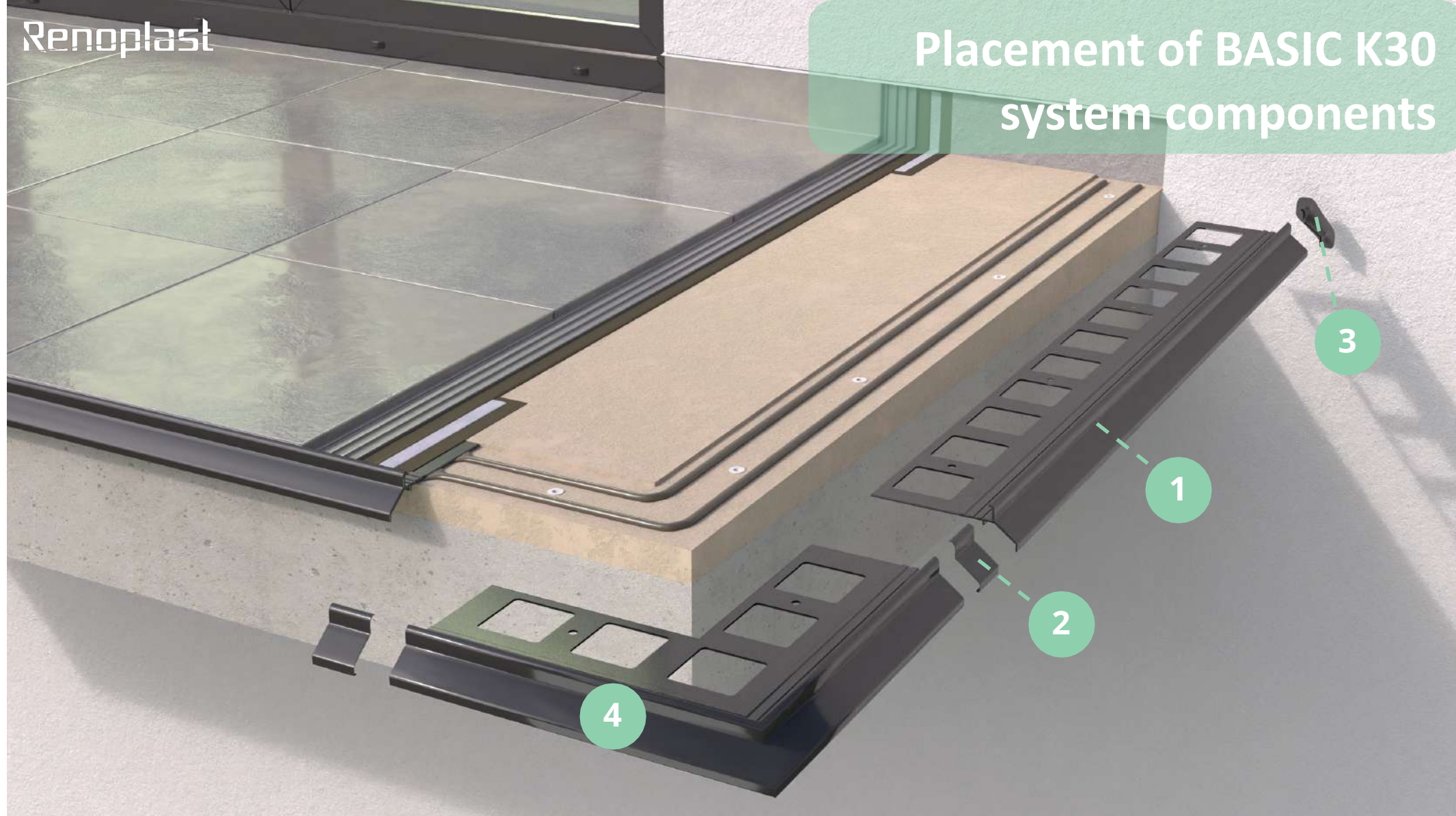
K30 drip edge 200 cm length
