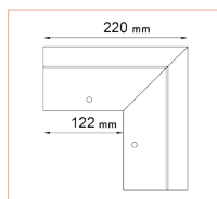
NZ K10R/90 NAROŻNIK ZEWNĘTRZNY
