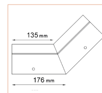
NW K10R/135 NAROŻNIK WEWNĘTRZNY
