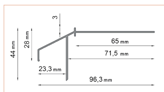
PROFIL PROSTY K10R
