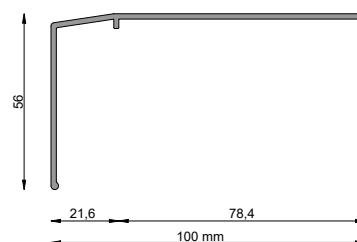
Profil okapowy prosty K301
