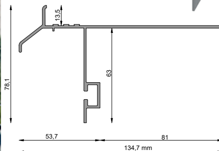
Profil okapowy prosty K40
