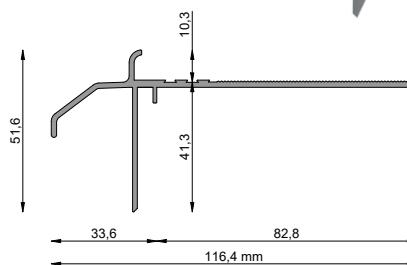
Profil okapowy prosty K20R
