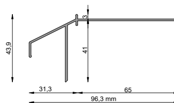
Profil okapowy prosty K100R
