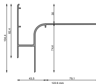
Profil okapowy prosty W30R PLUS
