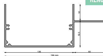
Koryto RENODRAIN
