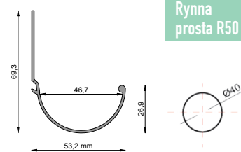
Przekrój rynny
