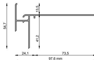
Profil okapowy prosty K35
